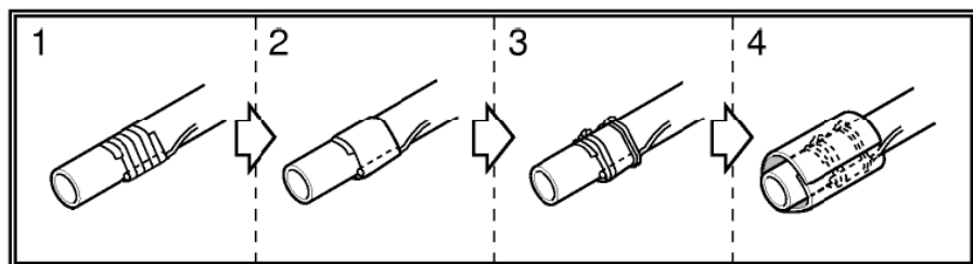
Obr.7 – UMÍSTĚNÍ SENZORU TEPLoty DO POTRUBÍ VZT
