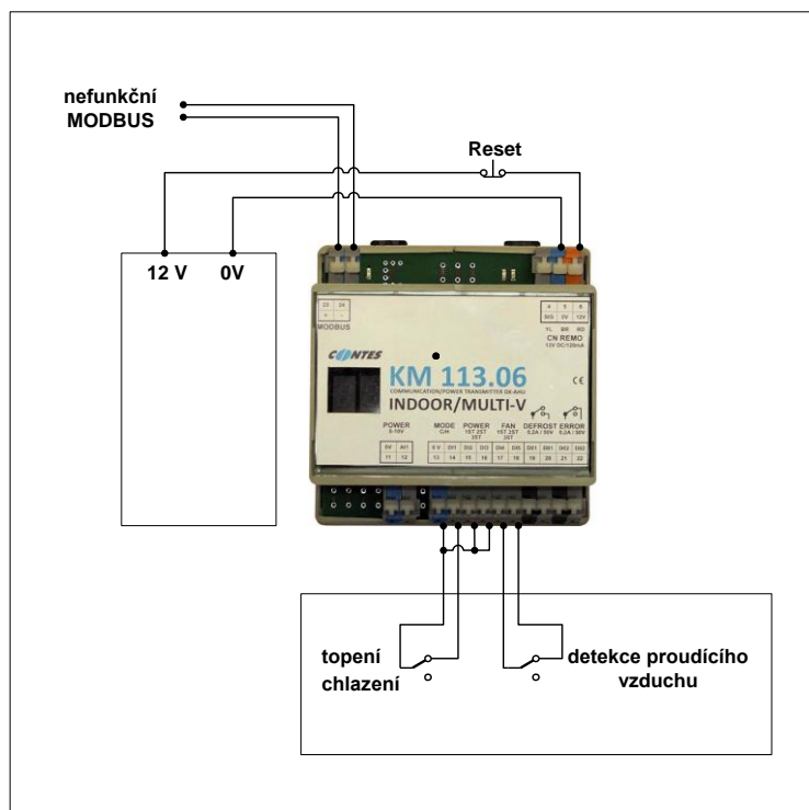
Obr.14 – SCHÉMA LOKÁLNÍHO OVLÁDÁNÍ V PŘÍPADĚ DOČASNĚ NEFUNKČNÍHO NADŘÁZENÉHO SYSTÉMU
