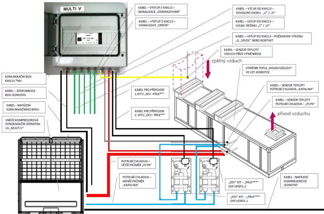
SCHÉMA ZAPOJENÍ KOMUNIKAČNÍHO BOXU KM113MV2 + EEV "PRLK048" V SYSTÉMU „KOMPRESOROVÁ JEDNOTKA MULTI V– JEDNOTKA VZT“
