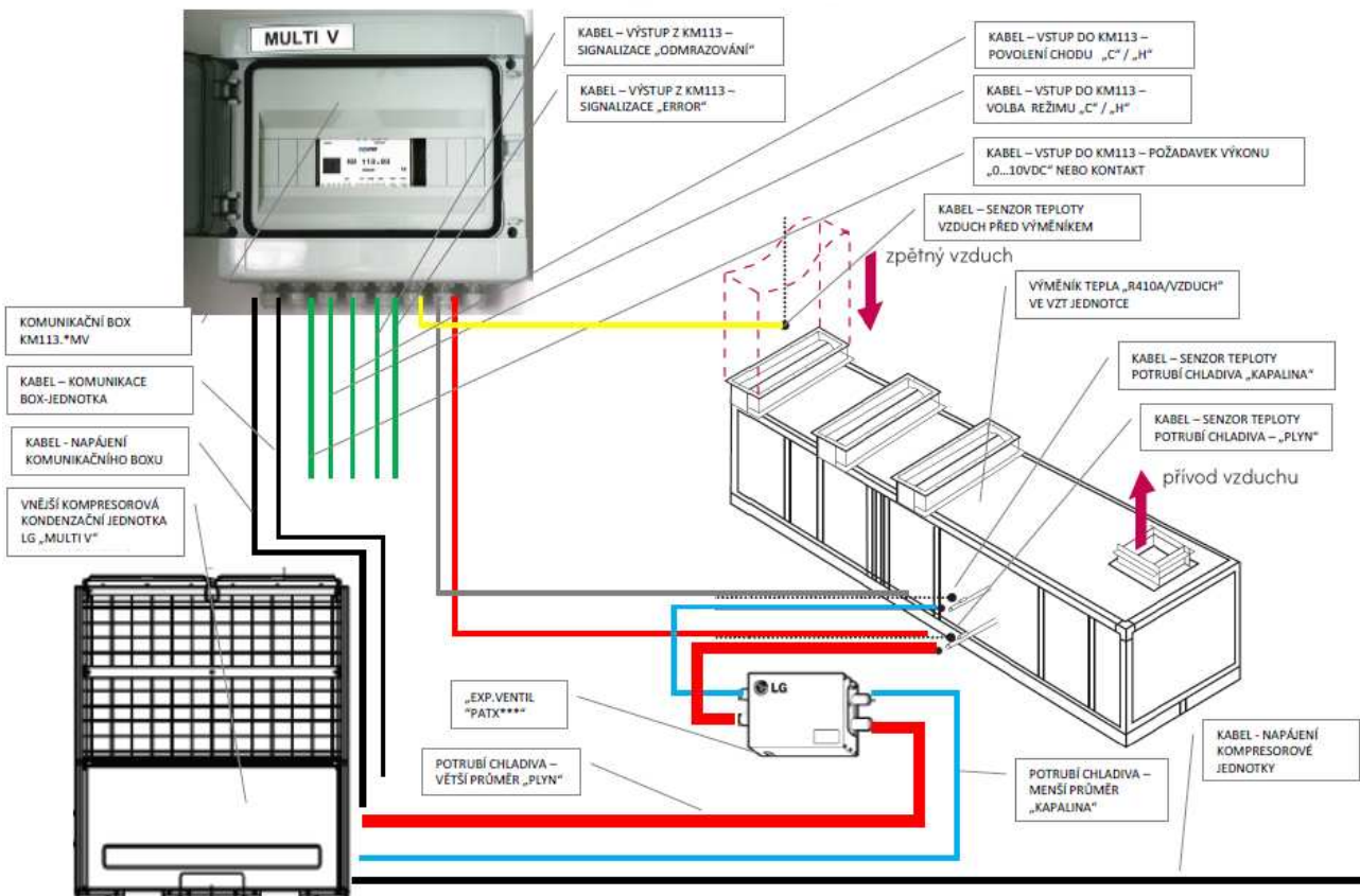
SCHÉMA ZAPOJENÍ KOMUNIKAČNÍHO BOXU KM113MV2 + VENTIL „PATX***“ V SYSTÉMU „KOMPRESOROVÁ JEDNOTKA MULTI V– JEDNOTKA VZT“
