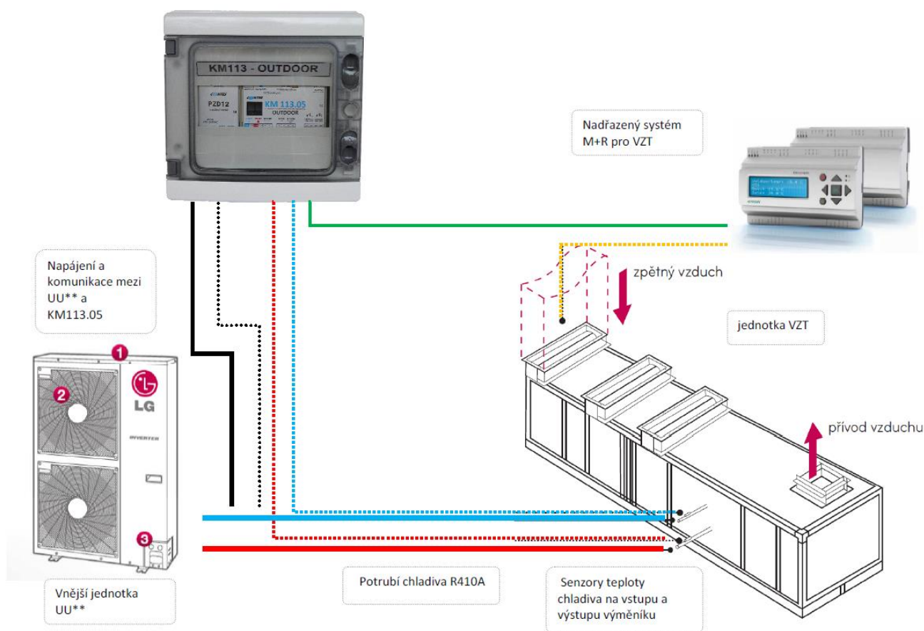
Obr.2 – CELKOVÉ SCHÉMA SVOREK
